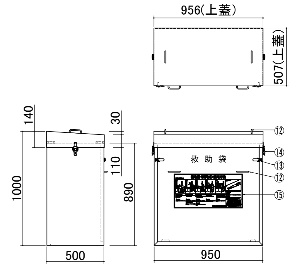
格納箱詳細図(S=1/20)A2時
