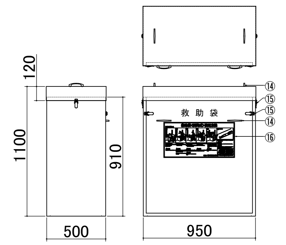
格納箱詳細図 (S=1/20) A2時
