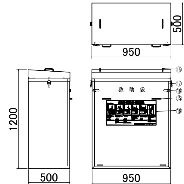
格納箱詳細図(S=1/20)A2時
